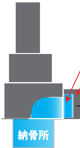
お墓の断面図
